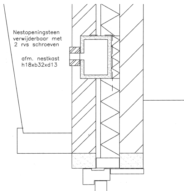
Tekening van een inbouwneestkast voor de gierzwaluw
